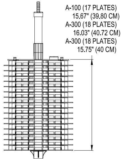
A100 - A600 12X20 CARTRIDGE
